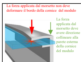
Figura 1 Forza applicata dal morsetto
